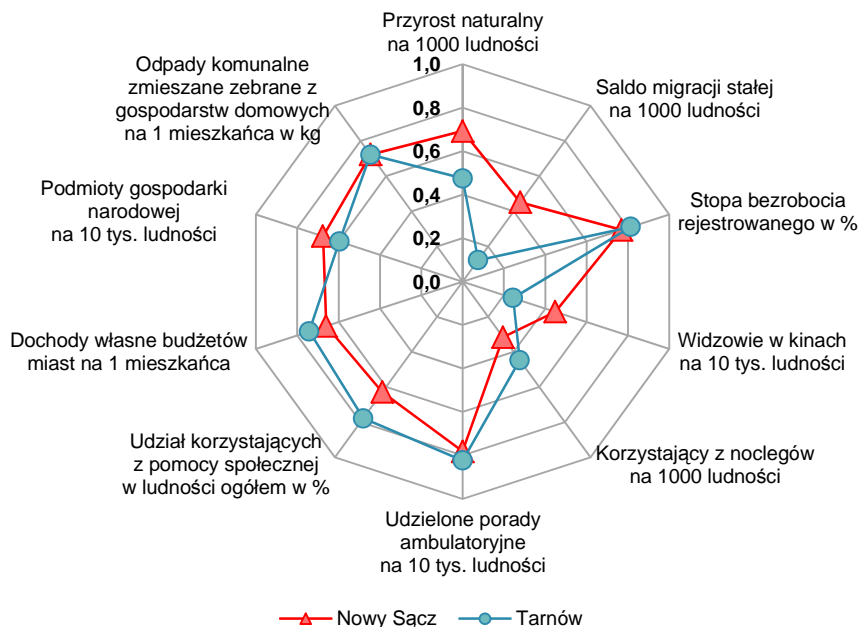
Wykr.24. Znormalizowane cechy diagnostyczne w 2013 r. (Nowy Sącz i Tarnów)
