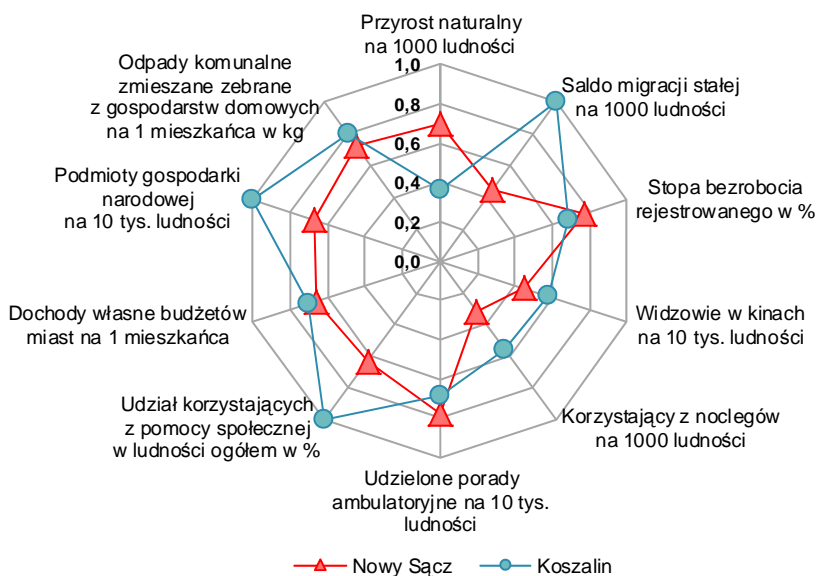
Wykr.22. Znormalizowane cechy diagnostyczne w 2013 r. (Nowy Sącz i Koszalin)
